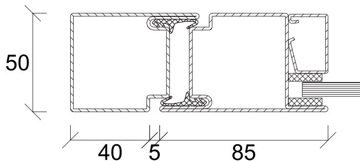
Jansen Economy 50 E30
