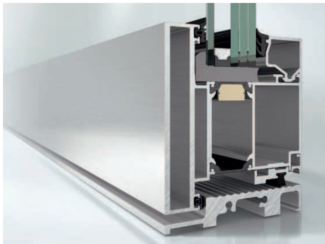
Schüco ADS 90 BR
