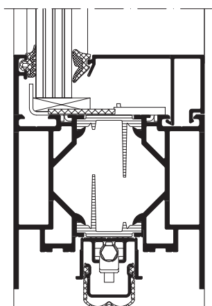
Schüco ADS 80 FR 30 lodret snit
