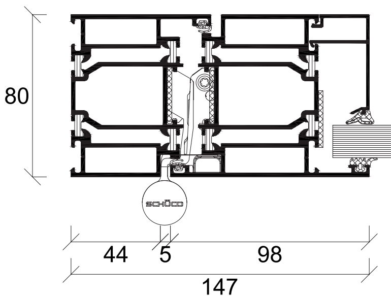
Schüco ADS 80 FR 30
