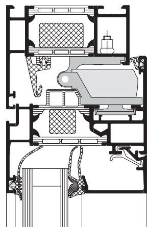
Vandret snit: Schüco vindue AWS 70.HI TipTronic
