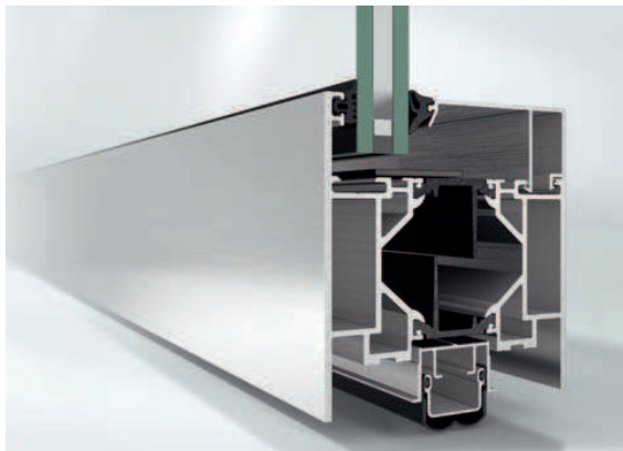
Schüco ADS 80 FR 30
