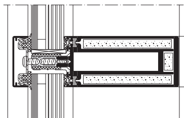
Schüco FW 50+ BF
