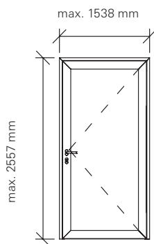
Schüco ADS 80 FR 60
