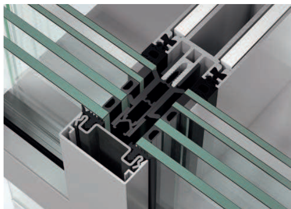
Højisoleret brandfacade Schüco FW 50+ BF
