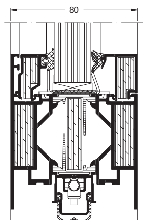
Schüco ADS 80 FR 60, bundsrit
