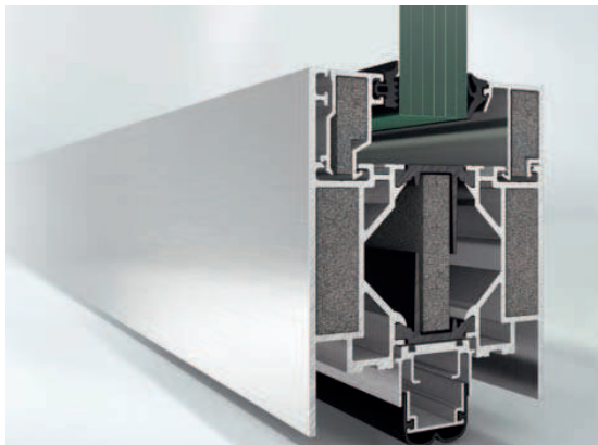
Schüco ADS 80 FR 60
