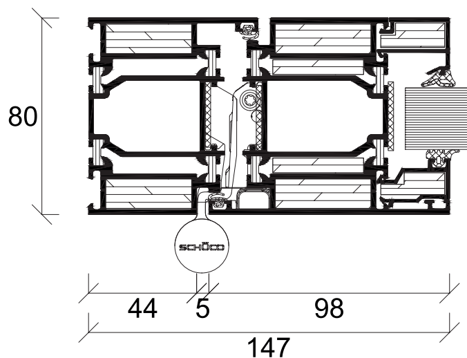
Schüco ADS 80 FR 60
